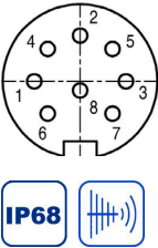
针脚定义
