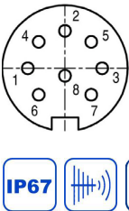
针脚定义
